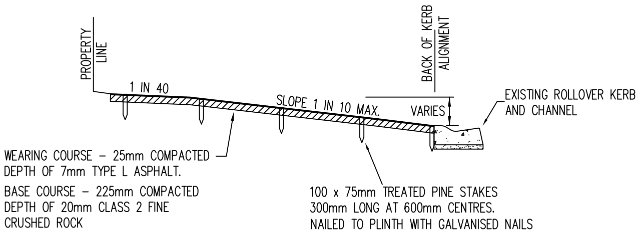
SECTION A-A
